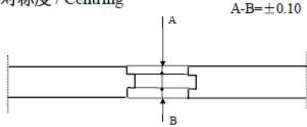
4.3.3 俯视图
