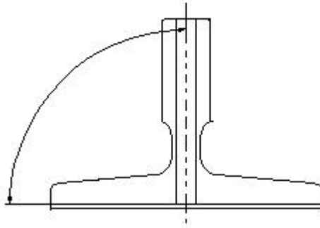
4.3.5 底面与侧面加工垂直度 90^\circ \pm 5'
