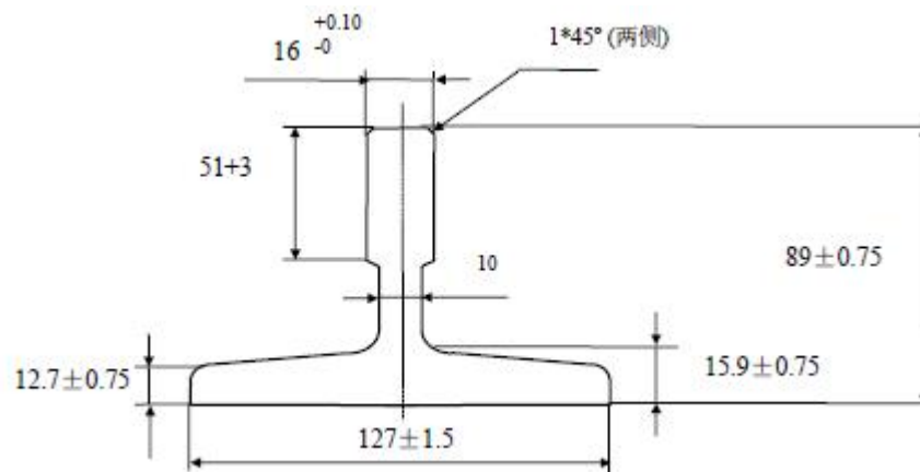
图 4.1.1 正视图
