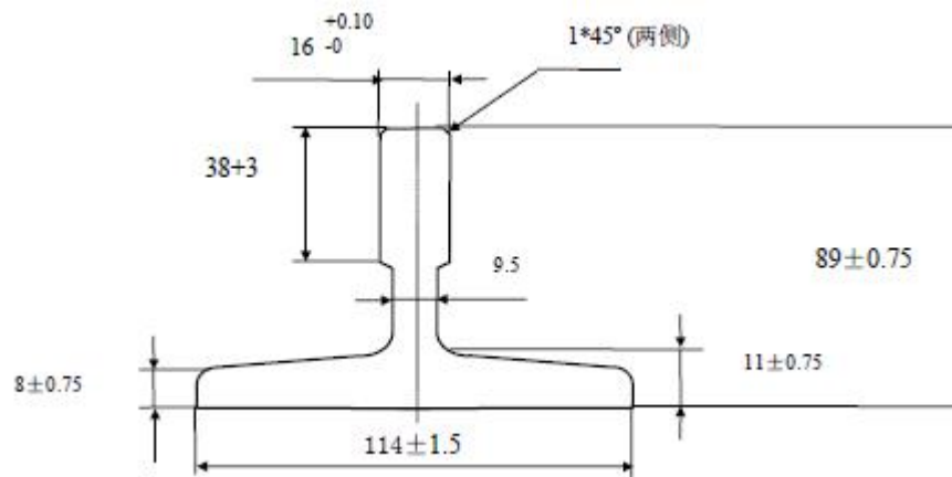
图 4.2.2 侧视图
