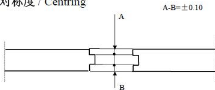
图 4.2.3 俯视图
