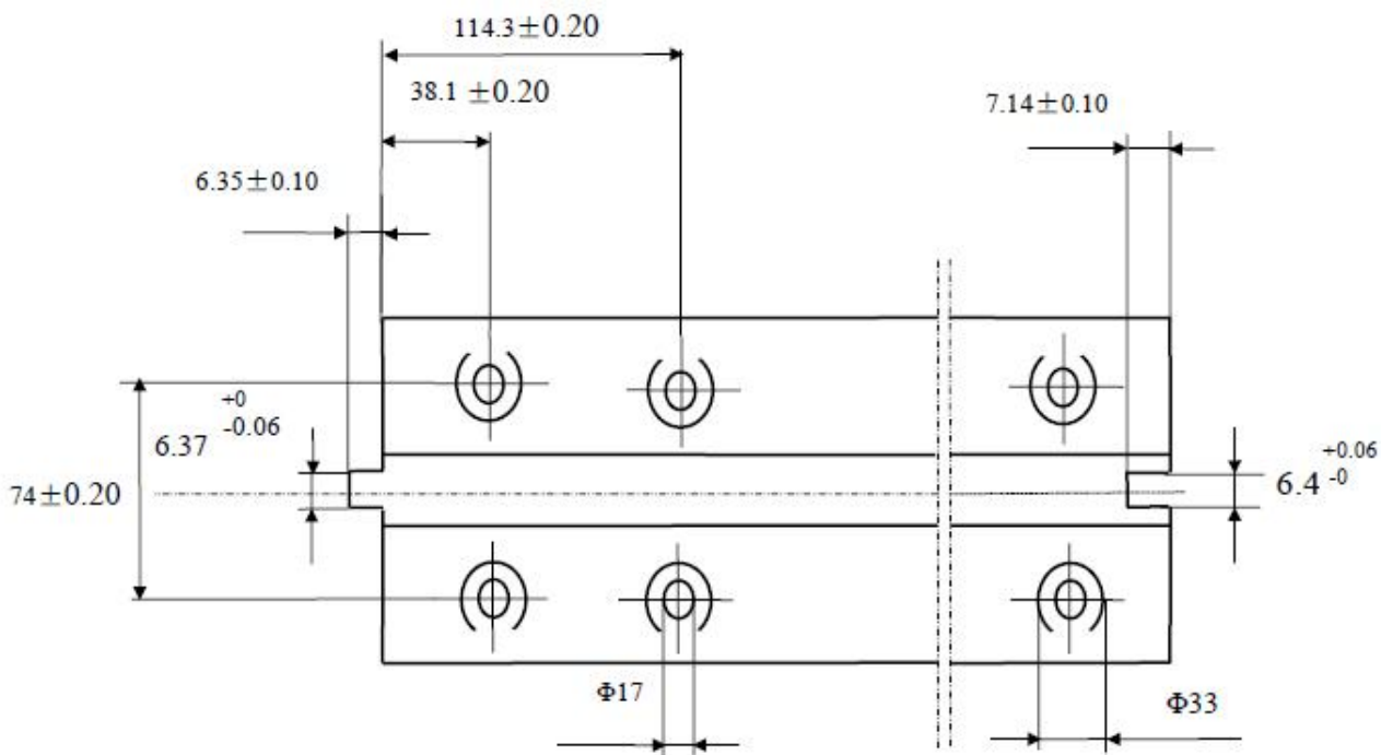
图 4.2.3 俯视图
