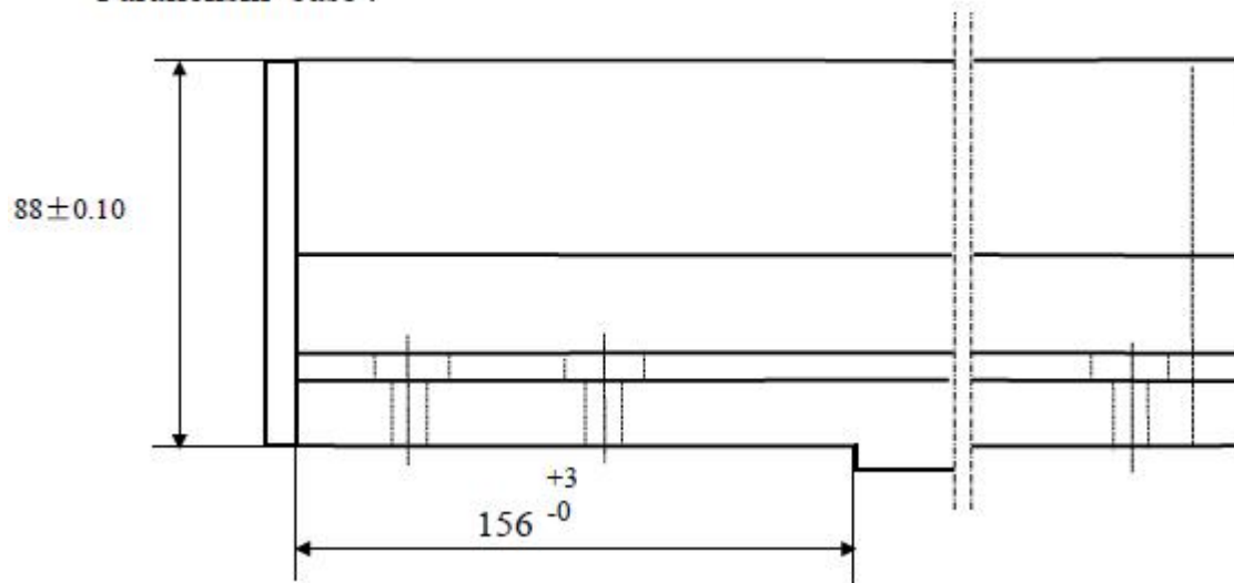
图 4.1.1 正视图
