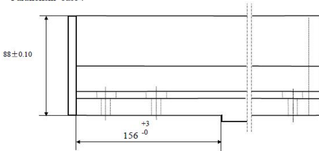
图 4.2.1 正视图
